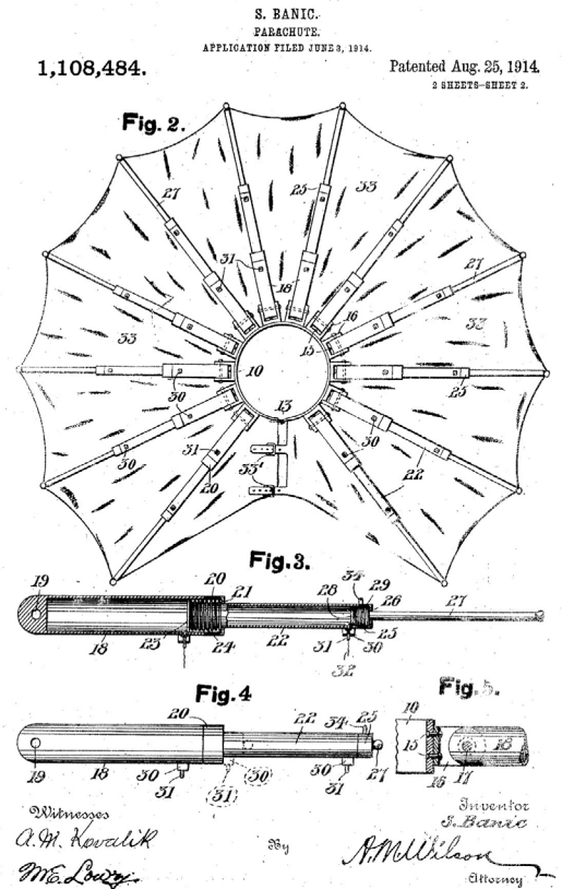
Nákres konštrukcie padáka, 1914
